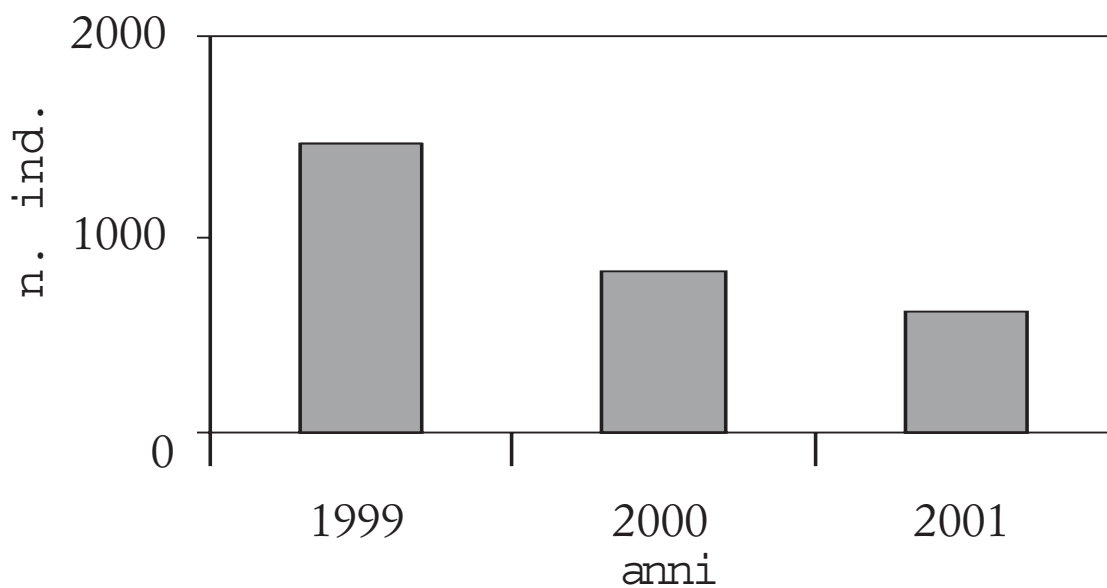
Fig 2 - Cormorano: numero di individui censiti durante il mese di gennaio.
