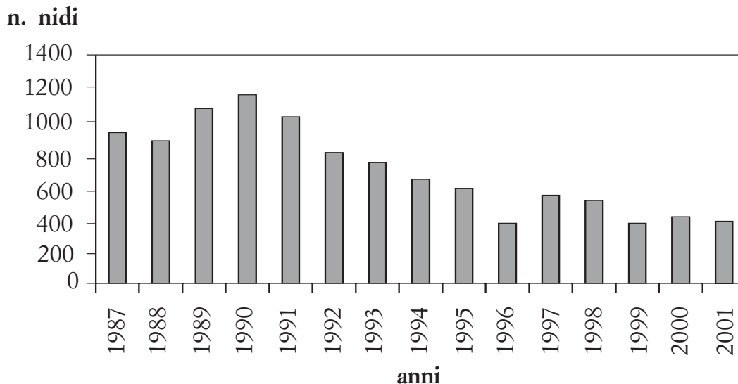
Fig. 4 - Numero nidi di nitticora censiti nelle colonie.
